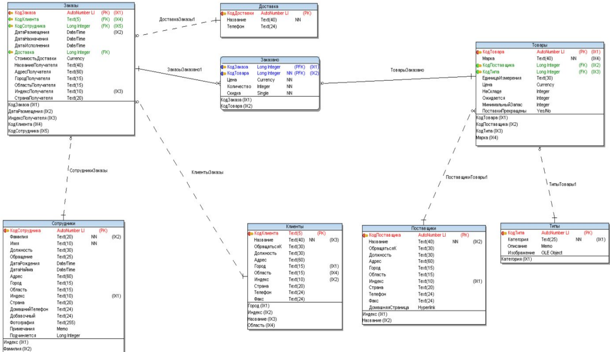
Рисунок 1 – Структура учебной базы данных «Борей».
